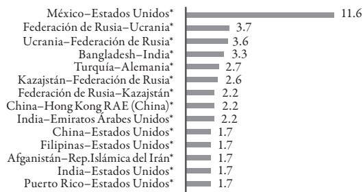
Principales corredores migratorios, 2010 Número de migrantes, millones
